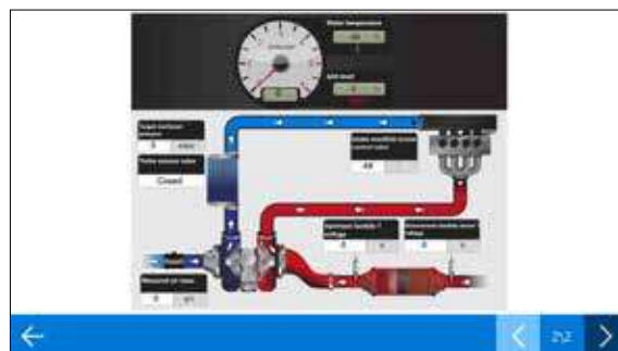
Sistema di dosaggio dell'agente riducente
